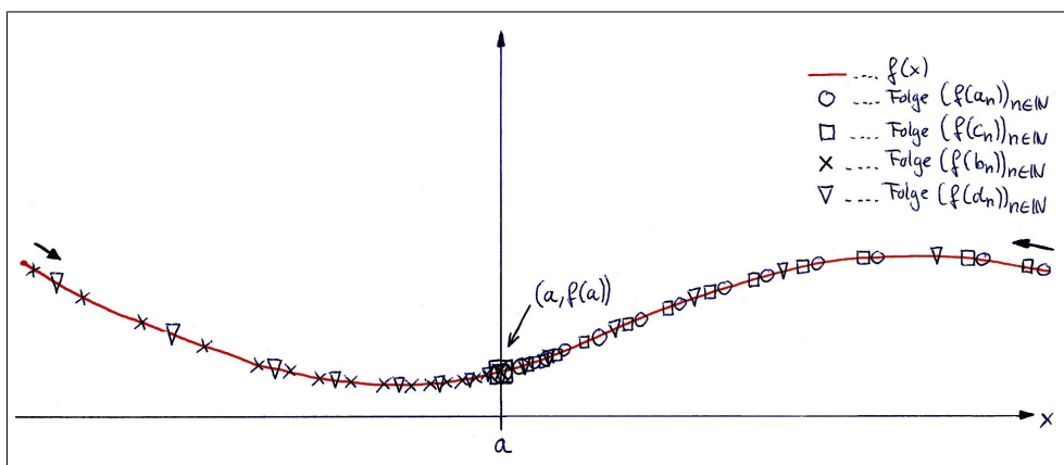
Abb. 2: Funktionsgrenzwert (a, f(a)) bei einer im Punkt a stetigen Funktion.
