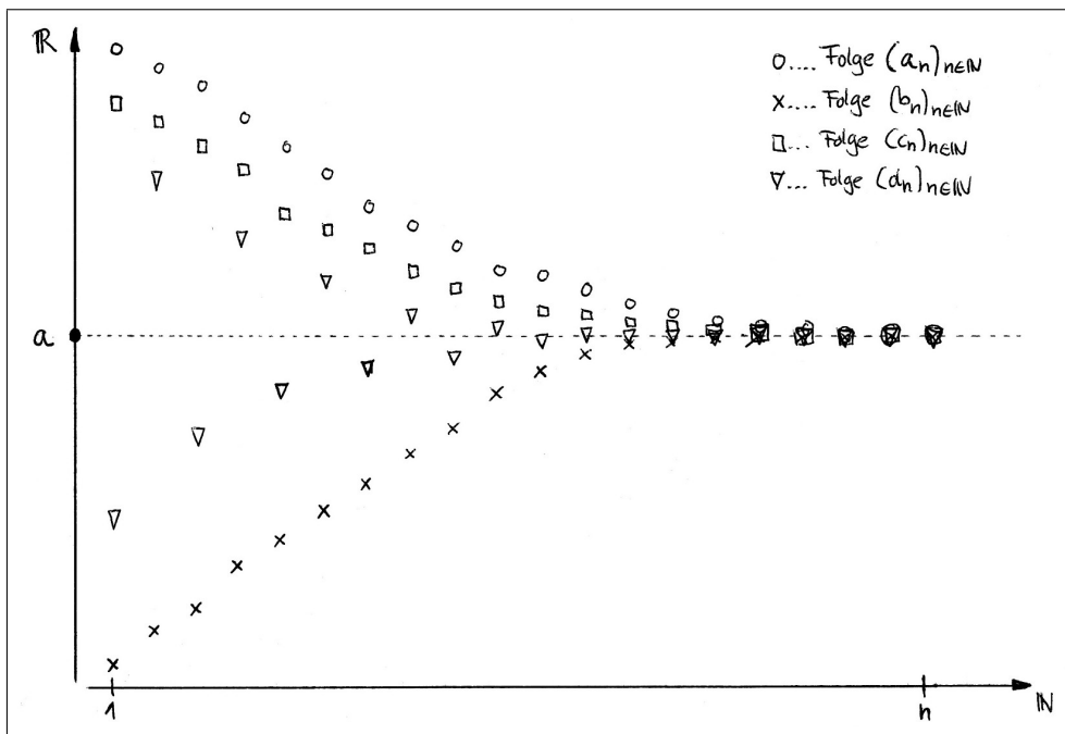
Abb. 1: Einige beliebig gewählte Folgen mit Grenzwert a
