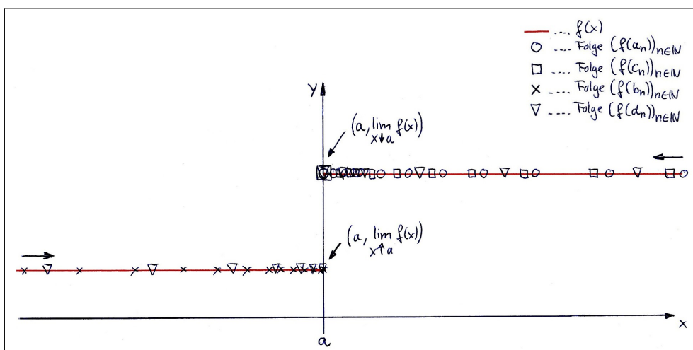
Abb. 3: Links- und rechtsseitiger Funktionsgrenzwert bei einer in a unstetigen Funktion.
