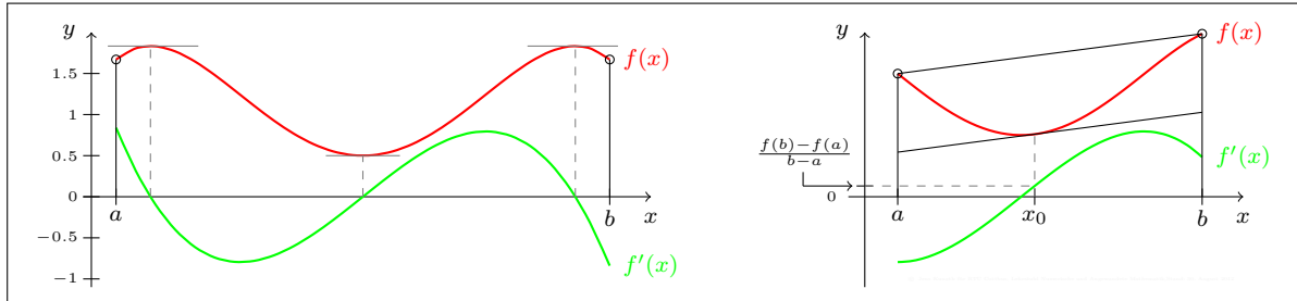
Abb. 2: Satz von Rolle (links) und Mittelwertsatz (rechts).
